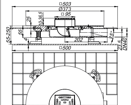
Geluidswerende afvoer CeraDrain Pure Plan, 100 x 100 mm
