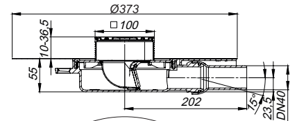
Vloerafvoer DalIDrain Select Plan OM, 100 x 100 mm
