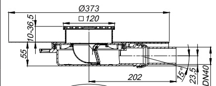
Vloerafvoer DalIDrain Pure Plan OM, 120 x 120 mm
