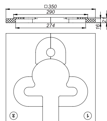
Montagehulp DallDrain Plan
