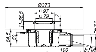
Vloerafvoer DallDrain Individual OM
