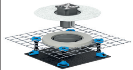
Geluidswerende afvoer CeraDrain Select, 100 x 100 mm
