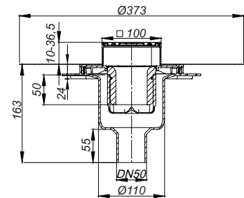
Vloerafvoer DallDrain Select verticaal OM, 100 x 100 mm
