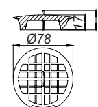
Haarzeef DallDrain GM
