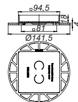
Opzetstuk DalIDrain natuursteen
