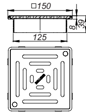
Opzetstuk DalIDrain Select Plus
