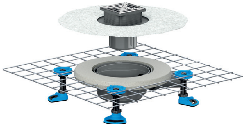
Complete set met afvoerkolk CeraDrain
