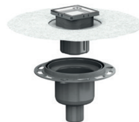
Vloerafvoer DallDrain Individual verticaal OM
