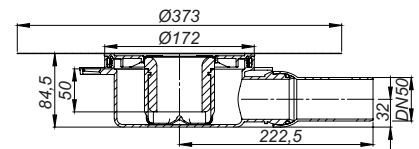
Afvoerkolk DallDrain
