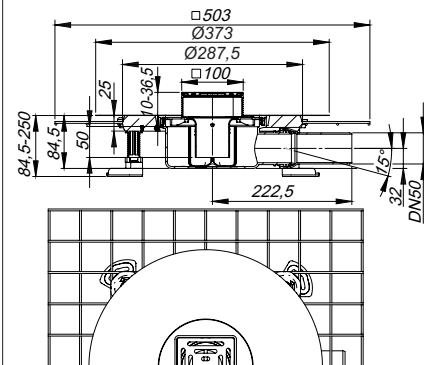
Vloerafvoer CeraDrain Select, 100 x 100 mm
