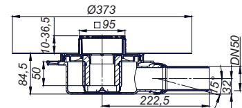
Vloerafvoer DallDrain Pure OM, 100 x 100 mm
