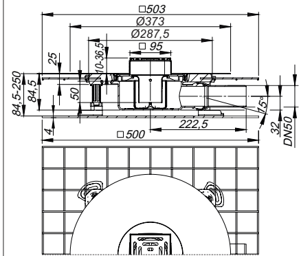
Geluidswerende afvoer CeraDrain Pure, 100 x 100 mm
