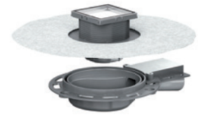
Vloerafvoer DallDrain Individual Plan OM
