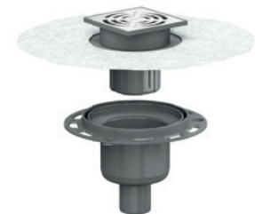
Vloerafvoer DallDrain Select verticaal OM, 120 x 120 mm
