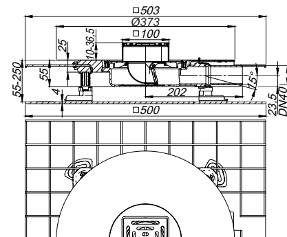
Geluidswerende afvoer CeraDrain Select Plan, 100 x 100 mm
