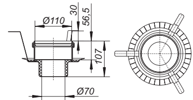
Brandwerend ruwbouwelement 2
