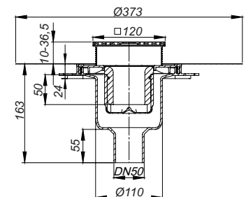
Vloerafvoer DallDrain Pure verticaal OM, 120 x 120 mm
