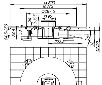
Vloerafvoer CeraDrain Pure 100 x 100 mm
