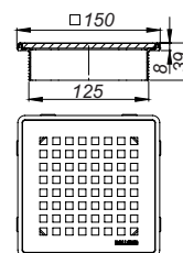
Opzetstuk DallDrain Select Quadra, 150 x 150 mm
