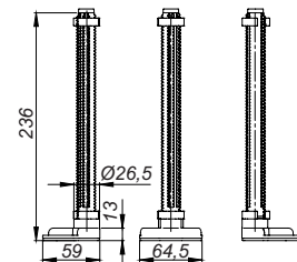
Montagevoeten DalIDrain
