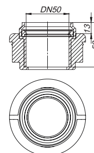
Badaansluiting DallDrain
