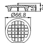
Haarzeef DallDrain
