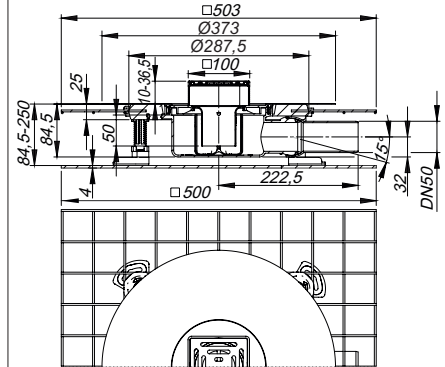
Geluidswerende afvoer CeraDrain Select, 100 x 100 mm
