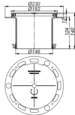
Opbouwelement DalIDrain
