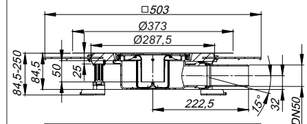
Afvoerkolk CeraDrain
