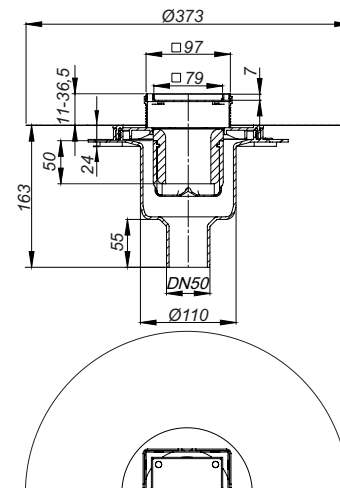
Vloerafvoer DallDrain Individual verticaal OM
