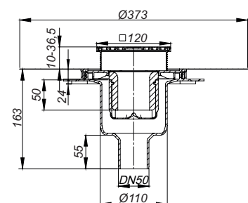
Vloerafvoer DallDrain Select verticaal OM, 120 x 120 mm
