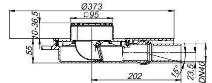
Vloerafvoer DalIDrain Pure Plan OM, 100 x 100 mm
