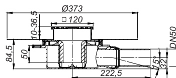
Vloerafvoer DallDrain Pure OM, 120 x 120 mm
