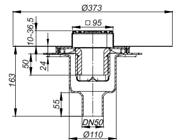
Vloerafvoer DallDrain Pure verticaal OM, 100 x 100 mm
