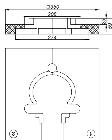
Montagehulp DallDrain
