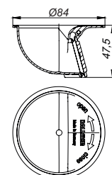
Mechanische stankafsluiter DalIDrain
