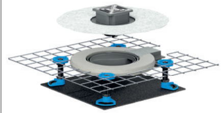
Geluidswerende afvoer CeraDrain Pure Plan, 100 x 100 mm
