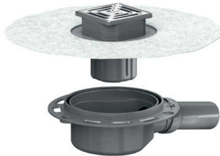
Complete set OM met afvoerkolk DallDrain
