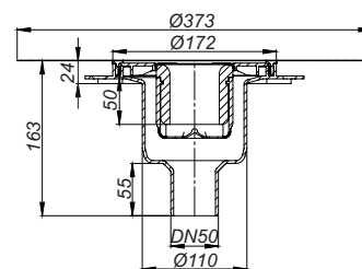
Afvoerkolk DallDrain verticaal
