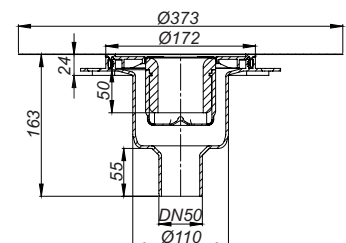
Afvoerkolk DallDrain verticaal
