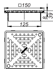
Opzetstuk DalIDrain Select RH
