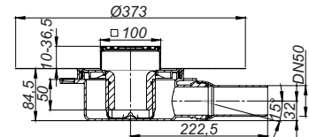
Vloerafvoer DallDrain Select OM, 100 x 100 mm
