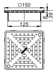
Opzetstuk DalIDrain Select Plus RH
