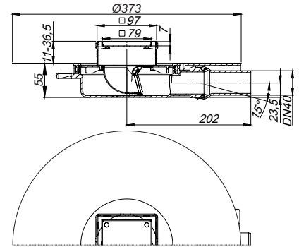
Vloerafvoer DallDrain Individual Plan OM
