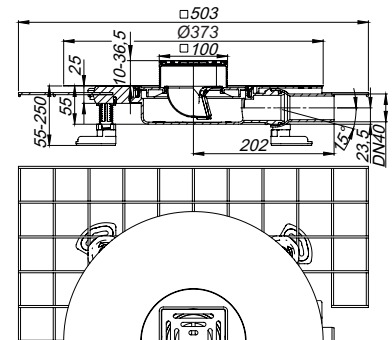
Vloerafvoer CeraDrain Select Plan, 100 x 100 mm
