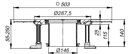
Opbouwelement CeraDrain Vario
